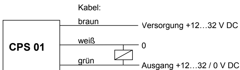
Belegung Stecker M8
